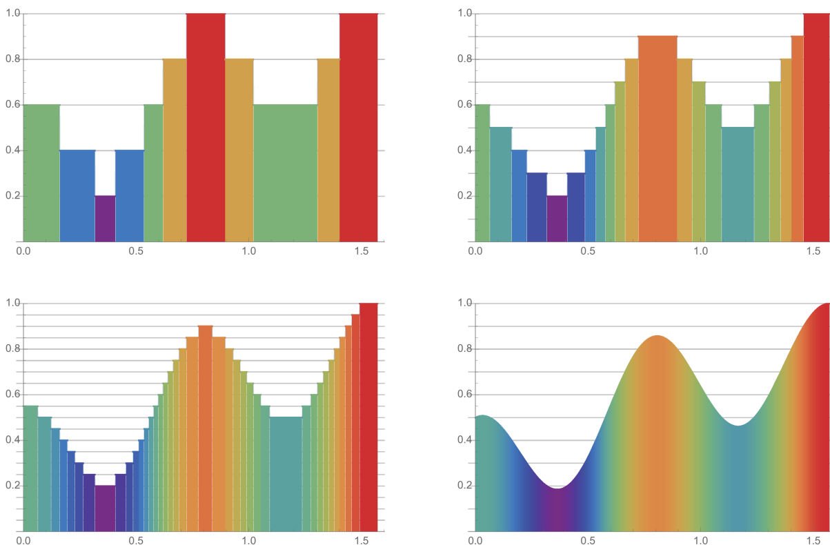
図 1.1: ルベーク積分では同じ高さ (色) の短冊をまとめて足しあげる。
