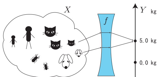
図 3.5: 写像のイメージ
