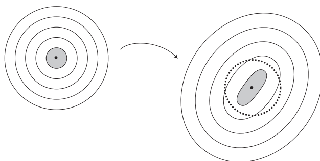
図 3.4: 距離空間における連続性のイメージ図．右の点線で囲まれた開球 B'(f(p), \epsilon) を定めると（どんなに小さくてもよい），像がそこに入るような開球 B(p, \delta) （灰色）を左で見つけることができる．
